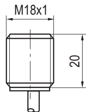
Габаритный чертеж
